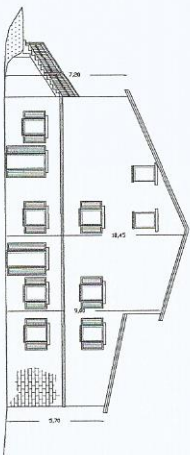
PROSPETTO NORD
